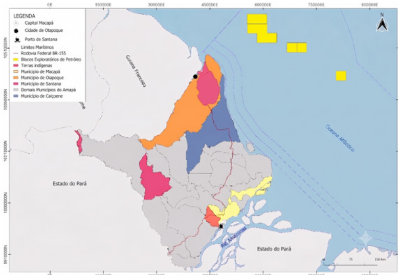
Mapa 1 - Mapa do Amapá com os municípios de Macapá, Oiapoque e Santana e os blocos da Margem Equatorial. Fonte: Dados IBGE, ANA, Marinha. Sistema projetado de coordenadas, SIRGAS 2000/UTM Zone 225. Organização: Tostes. Elaboração: Dário Júnior.
